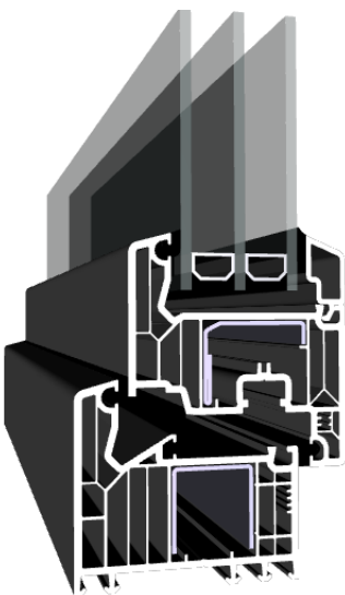
Normál ablak tok-szárny metszete
